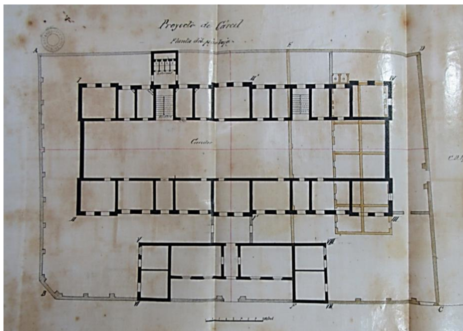
Segundo proyecto para cárcel pública elaborado por Bernardo Rígoli (1883) en Archivo General de la Provincia de Entre Ríos. Fondo Gobierno – Serie XIV J – Caja N°2 – Legajo N°5
