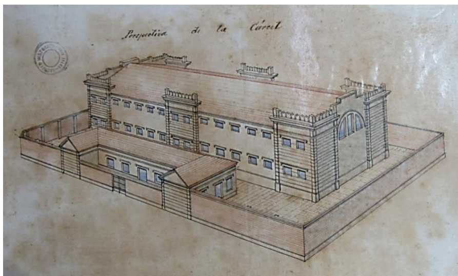
Axonometría del segundo proyecto para cárcel pública elaborado por Bernardo Rígoli (1883) en Archivo General de la Provincia de Entre Ríos. Fondo Gobierno – Serie XIV J – Caja N°2 – Legajo N°5
