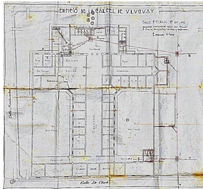
Plano Sanitario 28-10-1930 – Solicitud N°1800 – Archivo Obras Sanitarias – M.C.U.
