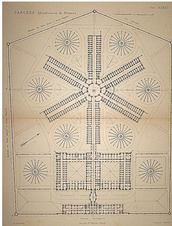
Comparación entre la planta de San Vittore en Milán, obra del Ing. Francesco Lucca y el proyecto de la Penitenciaría interprovincial de Bernardo Rígoli.
