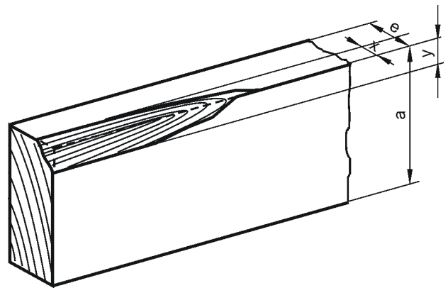
Figura 10 – Arista faltante
