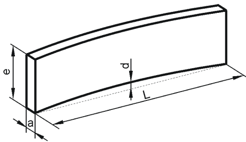
Figura 7 – Encorvado
