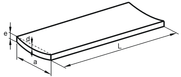
Figura 9 – Abarquillado
