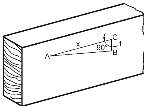
Figura 3 – Inclinación del grano
